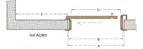
TEK KANAT KAPI GENİŞLİK ÖLÇÜLERİ
