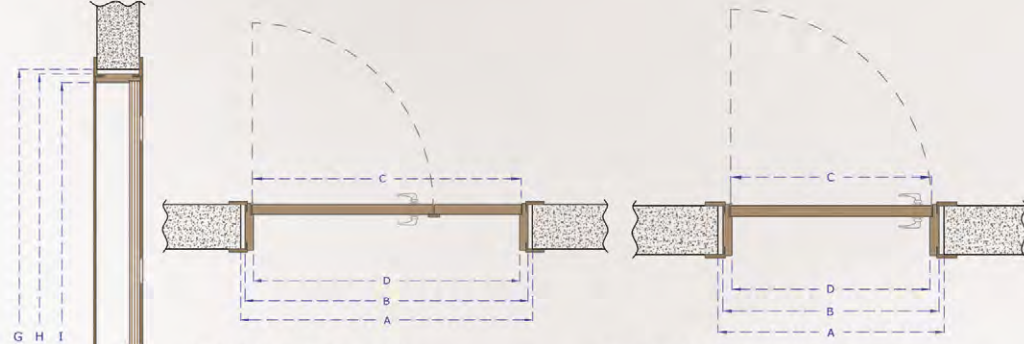
1.5 KANAT KAPI GENİŞLİK ÖLÇÜLERİ
