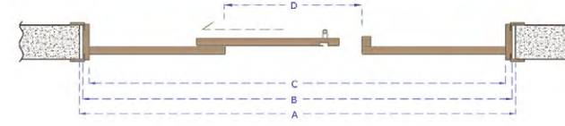
3 TAM KANATLI SÜRME KAPI GENİŞLİK ÖLÇÜLERİ
