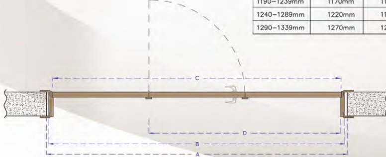
3 TAM KANATLI KAPI GENİŞLİK ÖLÇÜLERİ
