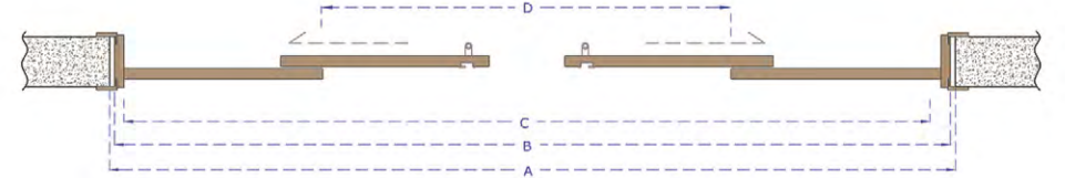
4 TAM KANATLI KAPI GENİŞLİK ÖLÇÜLERİ
