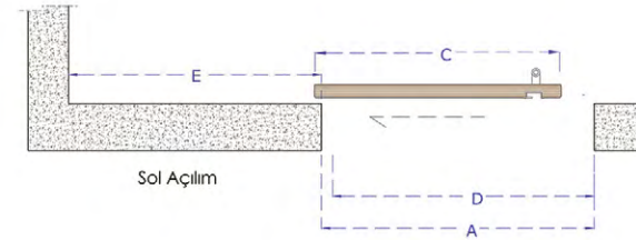
TEK KANAT KAPI GENİŞLİK ÖLÇÜLERİ
