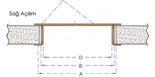
TEK KANAT GENİŞLİK ÖLÇÜLERİ
