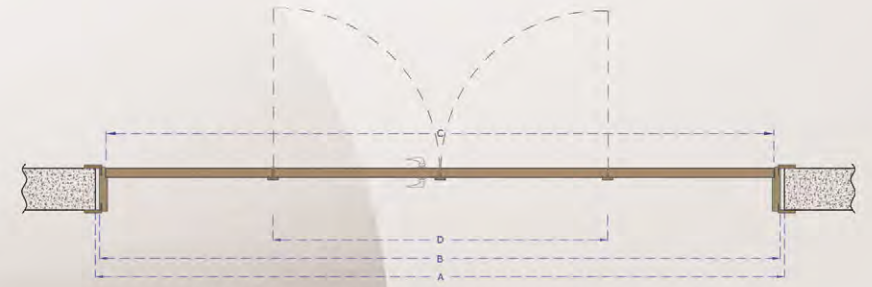
4 TAM KANATLI KAPI GENİŞLİK ÖLÇÜLERİ
