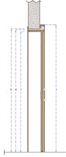
KAPI YÜKSEKLİK ÖLÇÜLERİ
