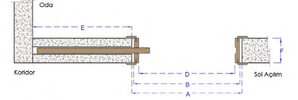
TEK KANAT KAPI GENİŞLİK ÖLÇÜLERİ
