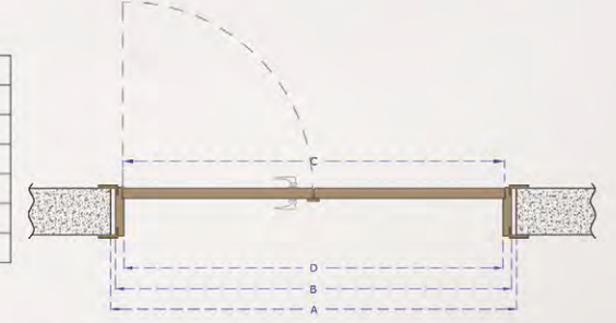
ÇİFT KANAT KAPI GENİŞLİK ÖLÇÜLERİ
