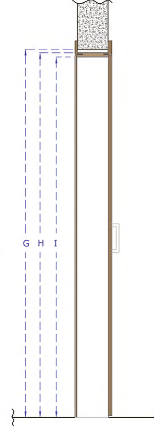
KATLANIR KAPAK BOY ÖLÇÜLERİ
