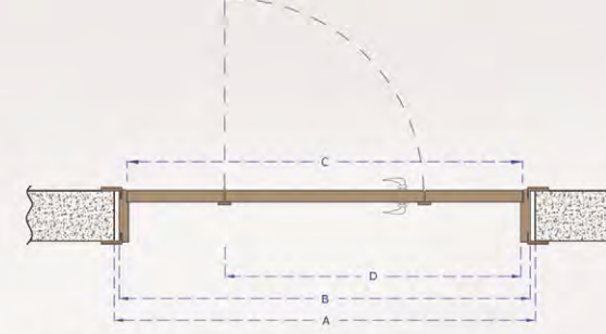
1 TAM 2 YARIM, 3 KANATLI KAPI GENİŞLİK ÖLÇÜLERİ
