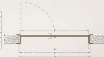
ÇİFT KANAT KAPİ GENİŞLİK ÖLÇÜLERİ
